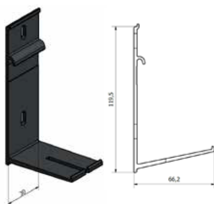
Uchwyt ML-119.02
